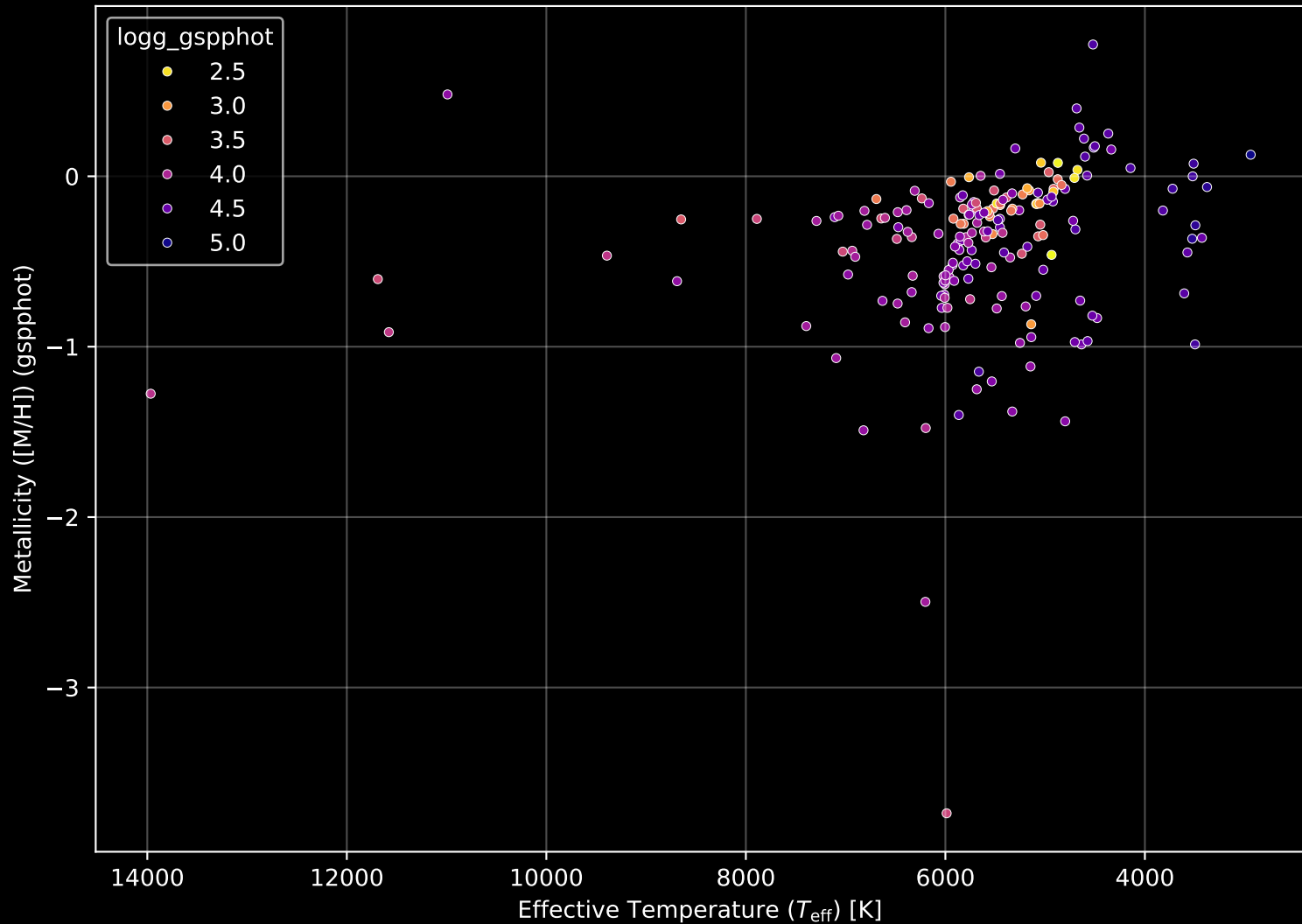
APOGEE DR17 Field: [K2_C13_183-16_btx] Stellar Population Parameters (n= 192)
